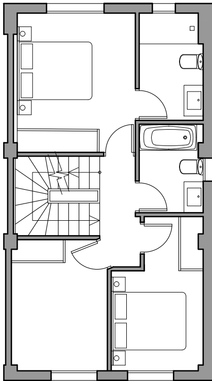
PLANTA PRIMERA
